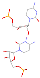
C:C pfS(sb:O2*-N3)
