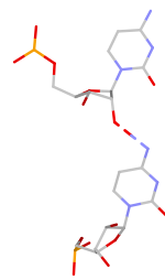
C:C pS(sb:O2*-N4)
