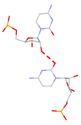
C:C fS(sb:O2*-O2)
