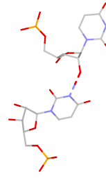
U:U pfS(sb:O2*-N3)
