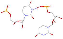
U:U S(bp:N3-O2P)
