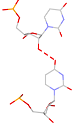
U:U pS(sb:O2*-O4)
