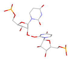
U:U pfS(sb:O2*-O2)
