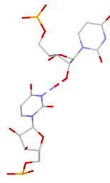
U:U fS(sb:O2*-N3)
