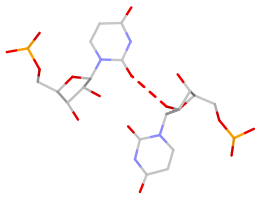
U:U rS(bs:O2-O2*)
