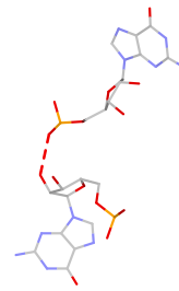
G:G rS(ps:O1P-O2*)_2
