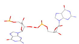
G:G rpS(ps:O2P-O2*)
