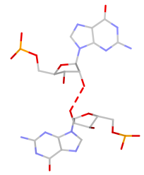
G:G rS(ss:O2*-O2*)_1
