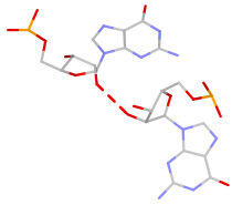
G:G rS(ss:O2*-O2*)_2
