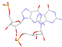
G:G pS(sp:O2*-O1P)
