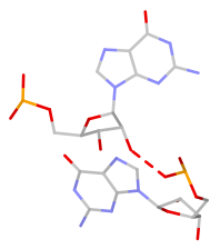
G:G S(sp:O2*-O2P)
