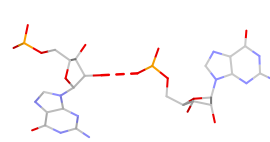
G:G rpS(ps:O1P-O2*)
