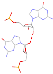
G:G S(ss:O2*-O2*)
