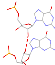
G:G pS(ss:O2*-O2*)
