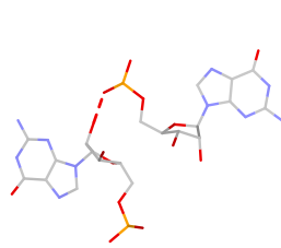
G:G rS(ps:O1P-O2*)_1
