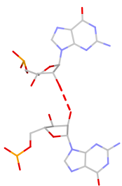
G:G rpS(ss:O2*-O2*)
